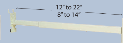
Adj. 3/4" PowerArm Pegboard PP-1222PB-34FFSL+(color) PP-814PB-34FFSL+(color)
